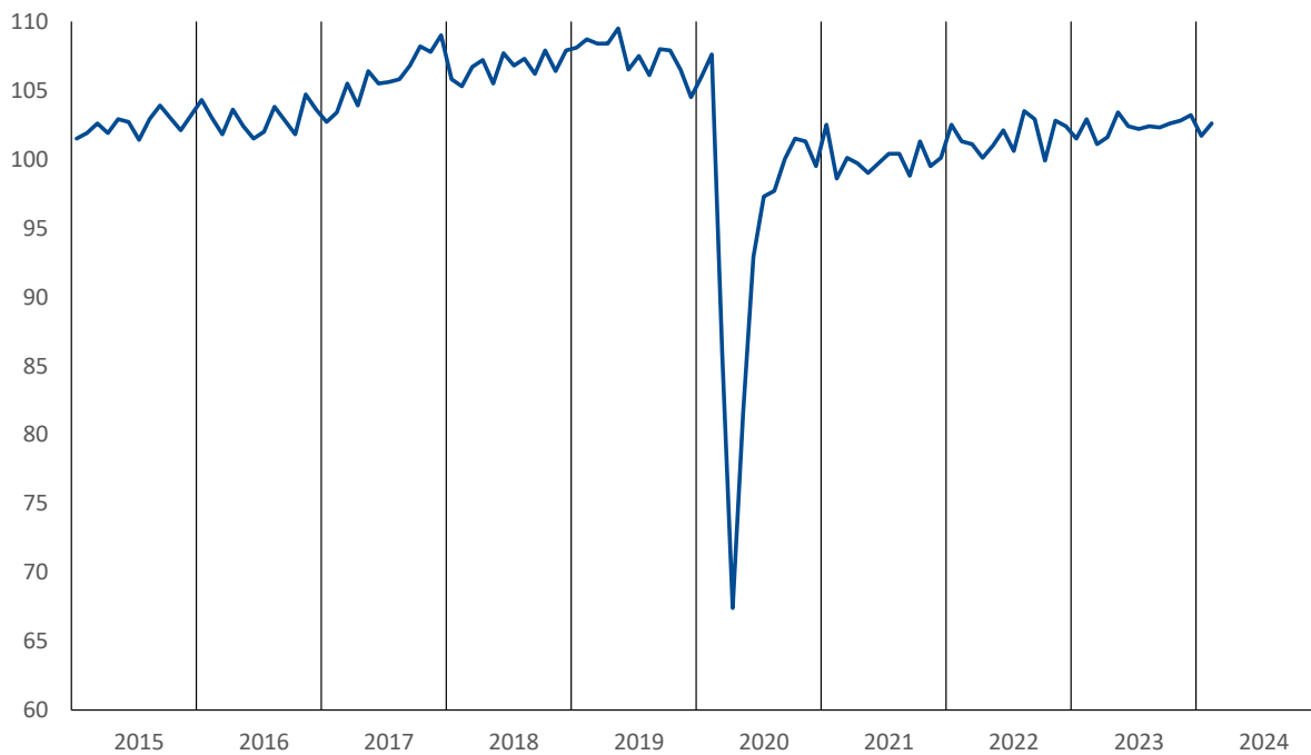
Industrieproduktion, saisonbereinigt, 2010 = 100
